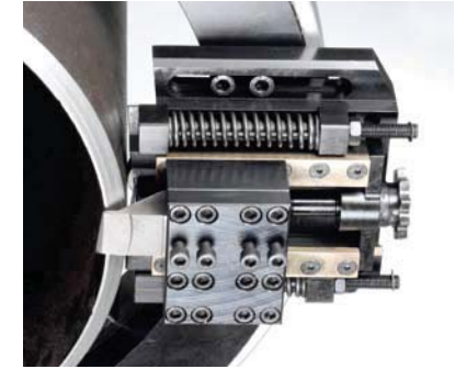
DISPONIBILI DUE PORTAUTENSILI CON SISTEMA COPIATURA DEL PROFILO DIAMETRO ESTERNO TUBO PER ELIMINARE DIFFERENZE DI SMUSSO DOVUTE ALL'OVALIZZAZIONE DEL TUBO.
